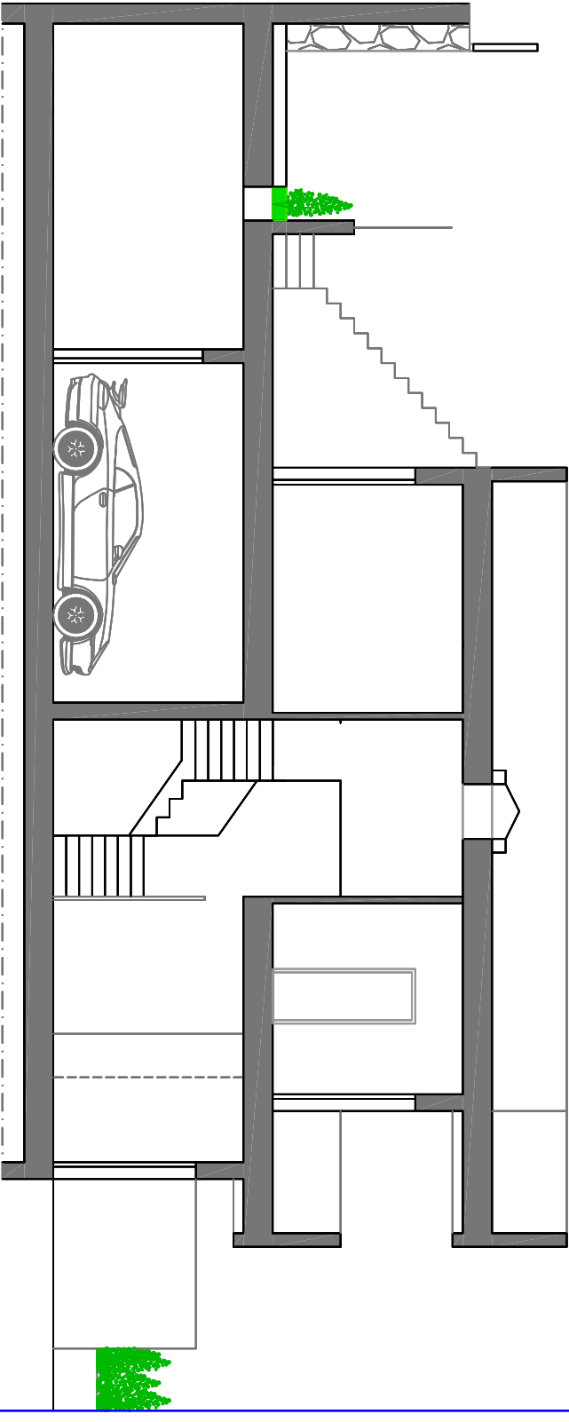
SECCIÓN LONGITUDINAL
