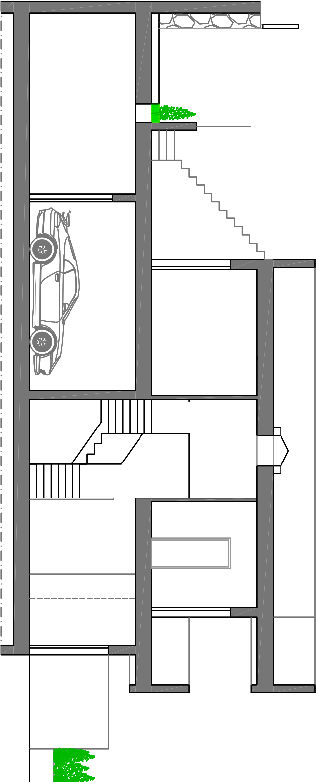
SECCIÓN LONGITUDINAL
