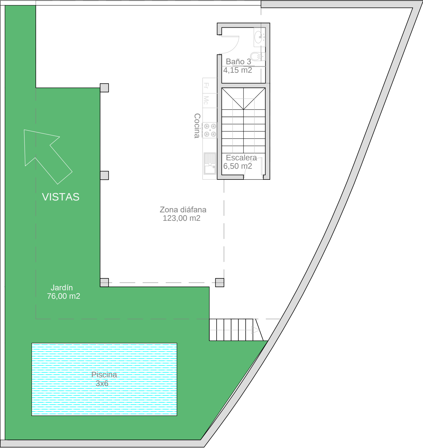
PLANTA BAJA
