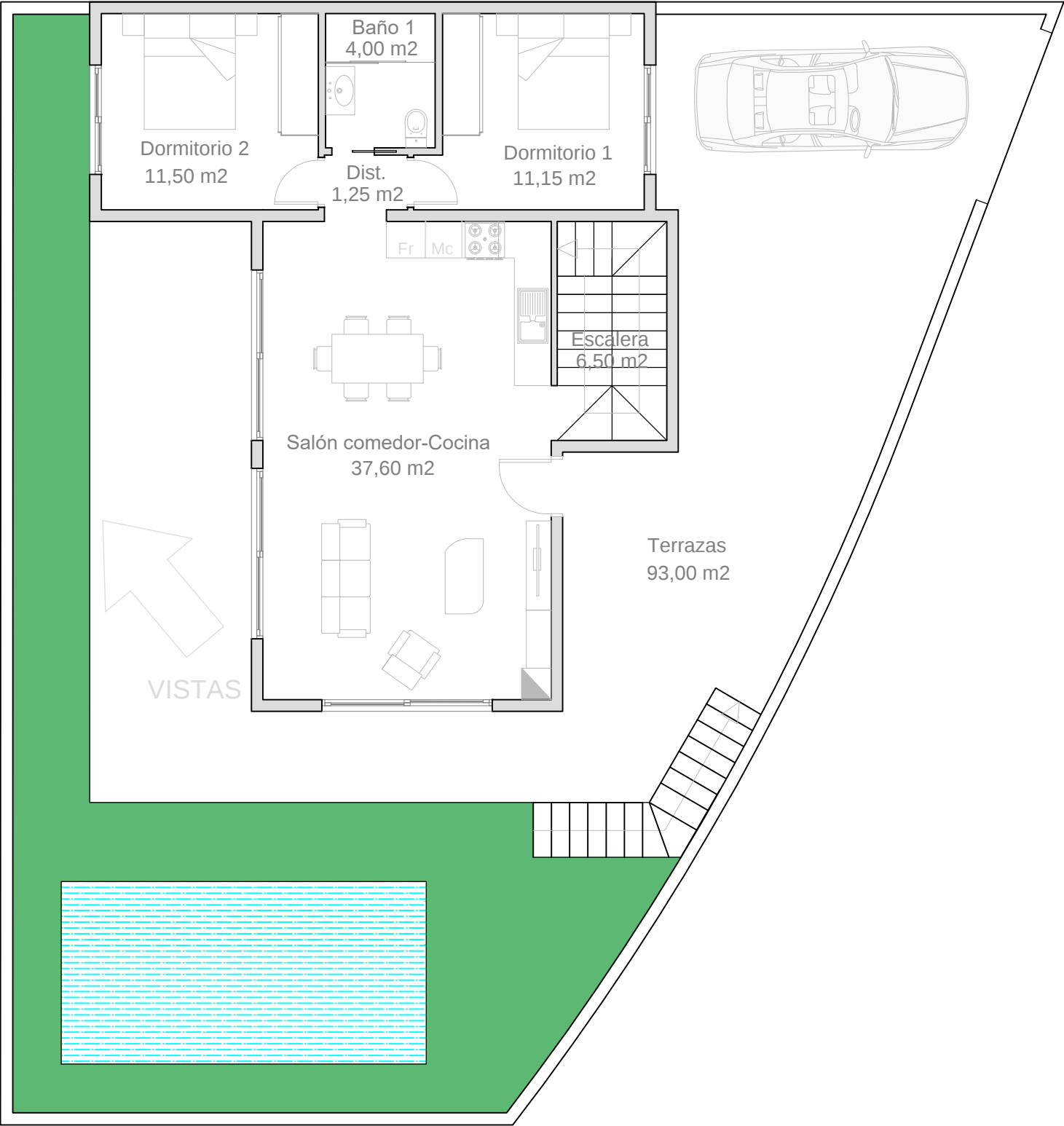
PLANTA INTERMEDIA
