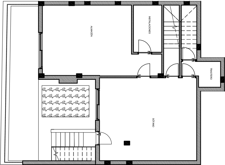
PLANTA SEMISÓTANO
