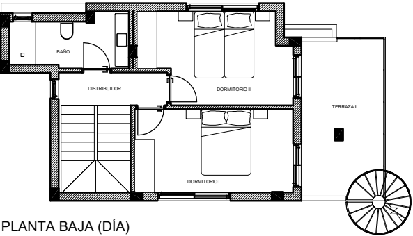
PLANTA BAJA (DÍA)
