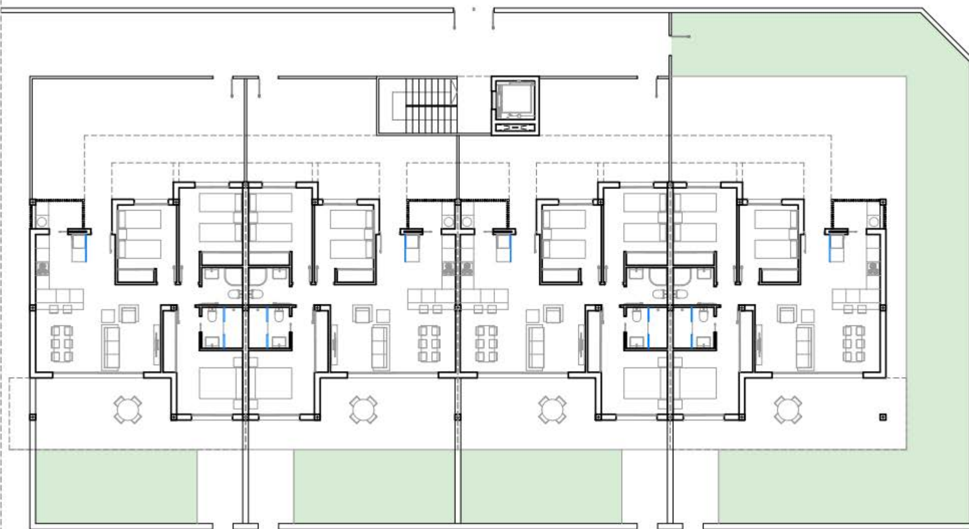
PLANTA BAJA
