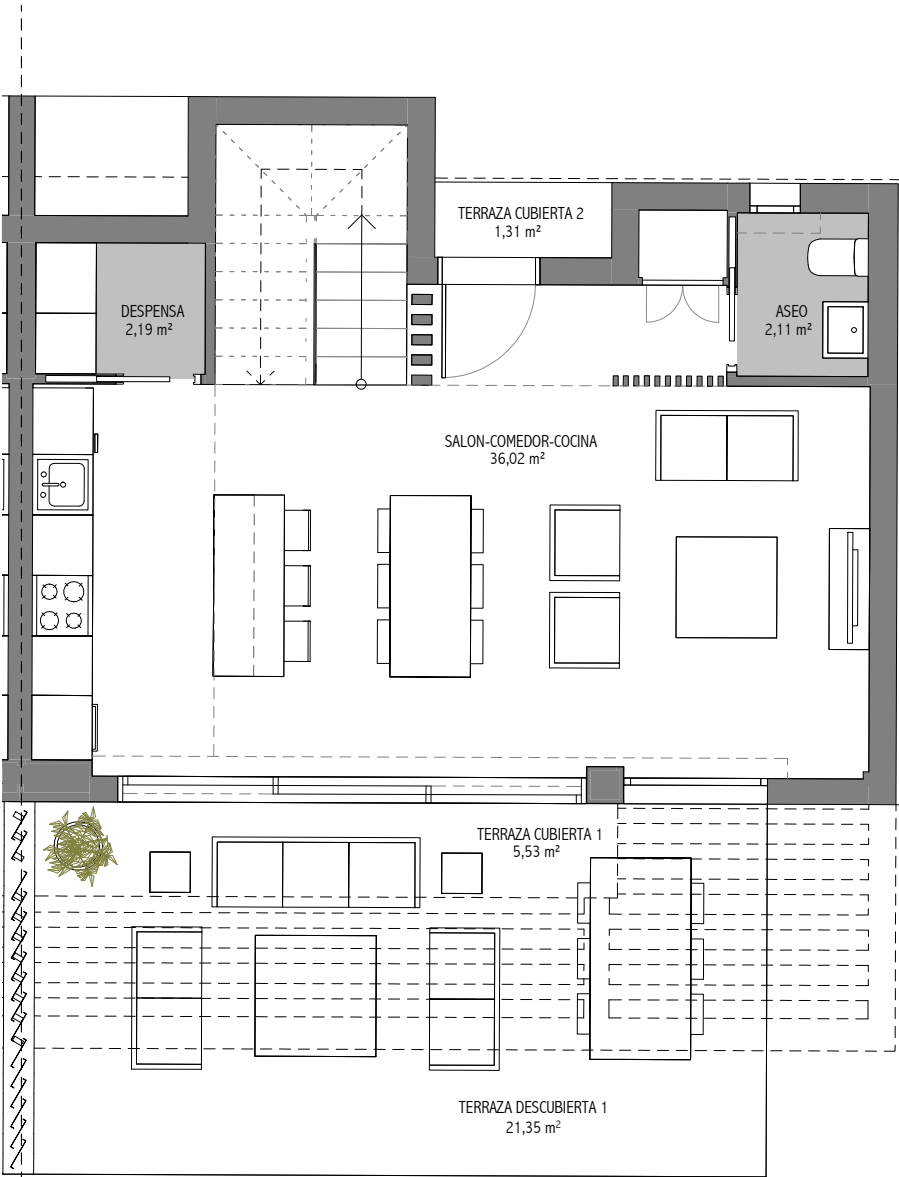
PLANTA BAJA 1:75
