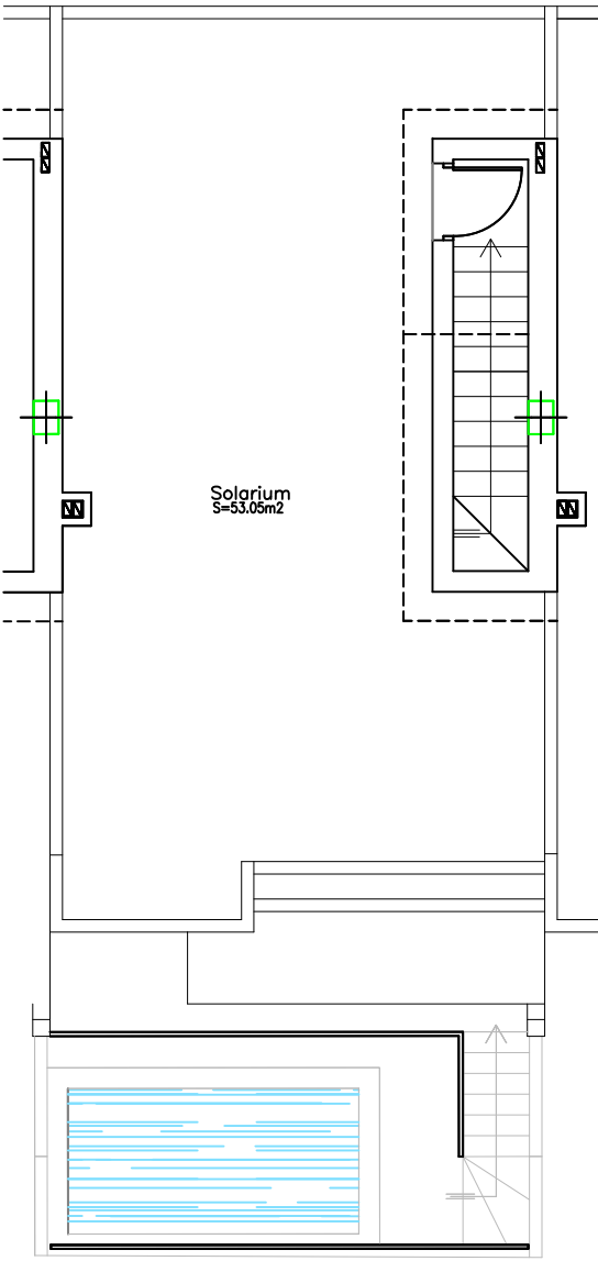
PLANTA SOLARIUM
