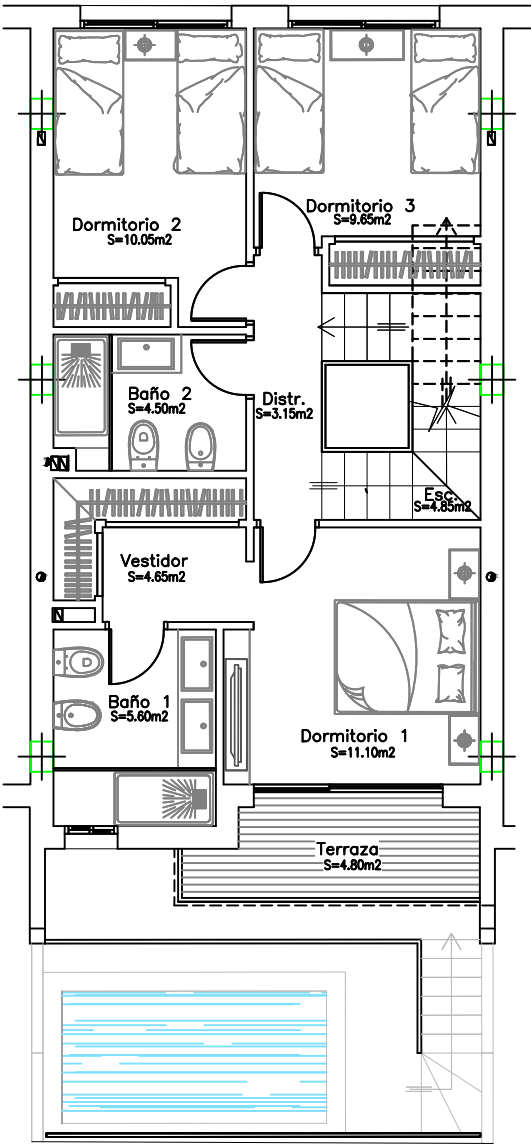
PLANTA ALTA
