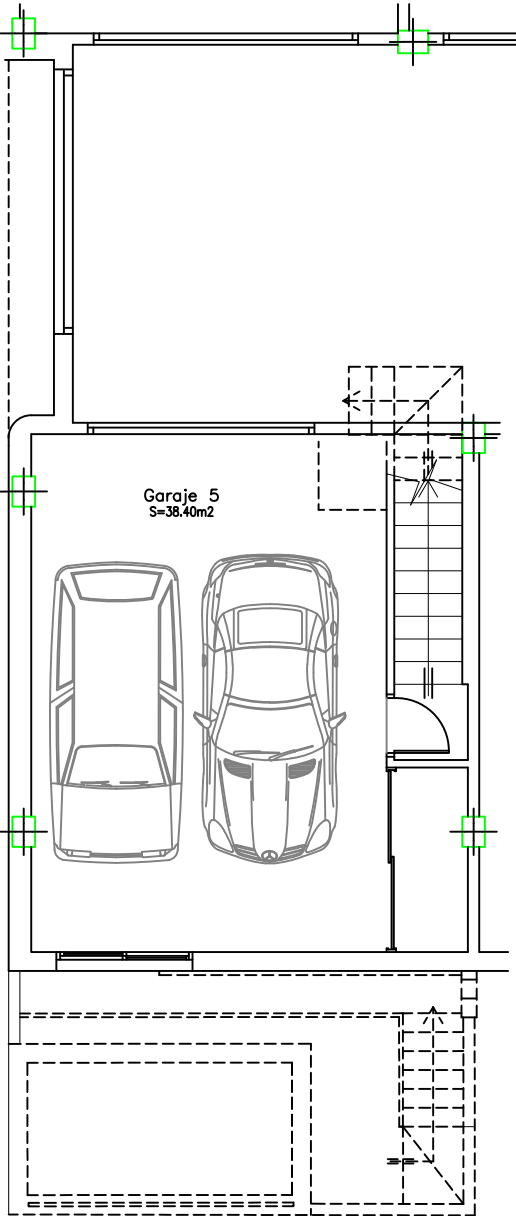
PLANTA GARAJES
