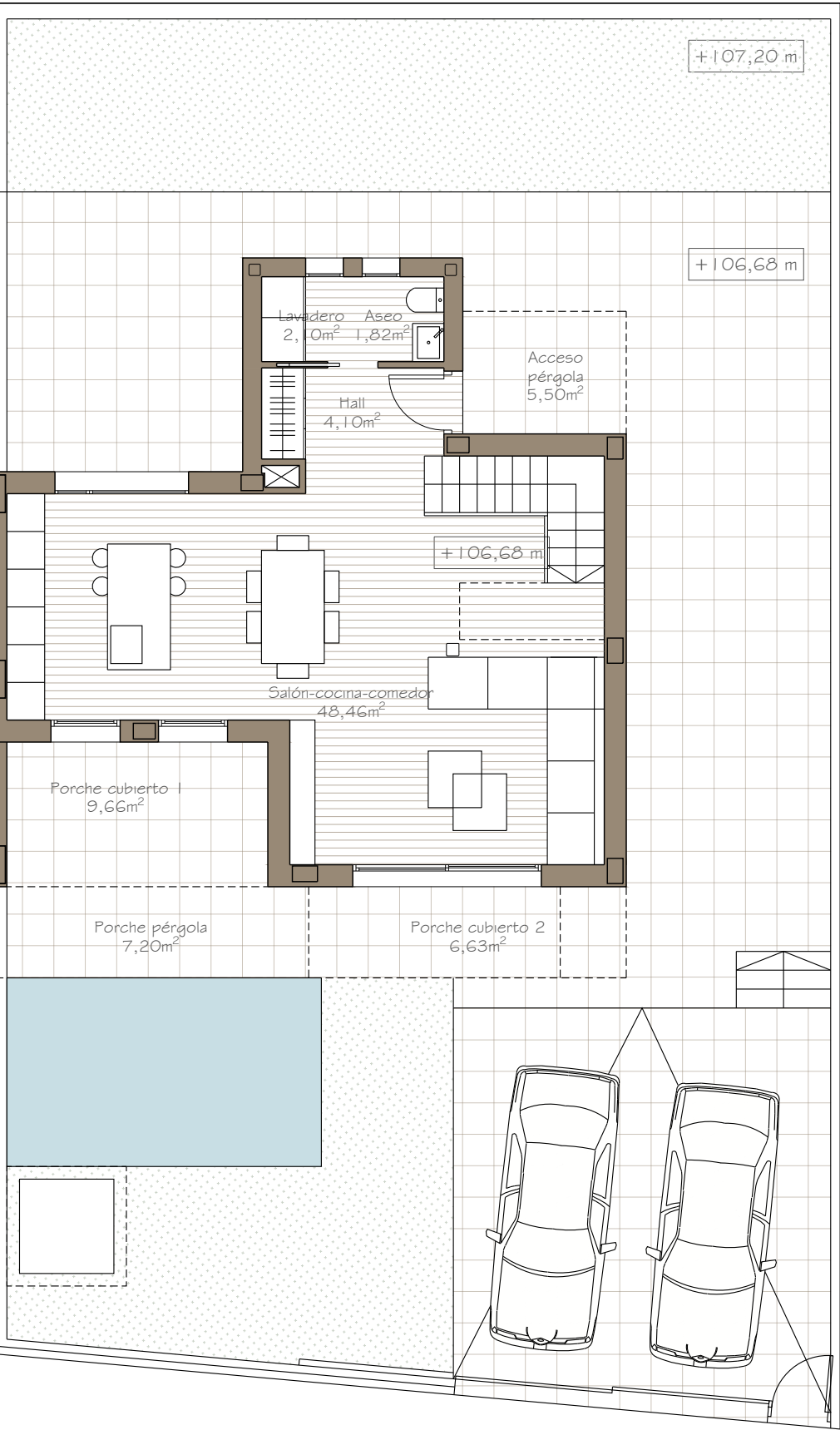
PLANTA BAJA
