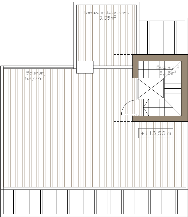
PLANTA CASTILLETE
