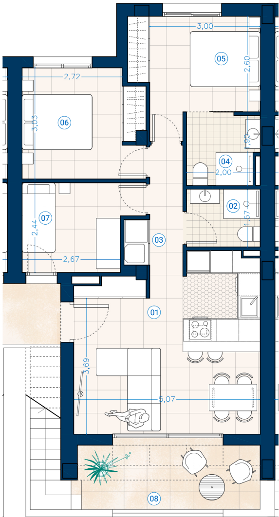
DIN A4 - e:1/100
