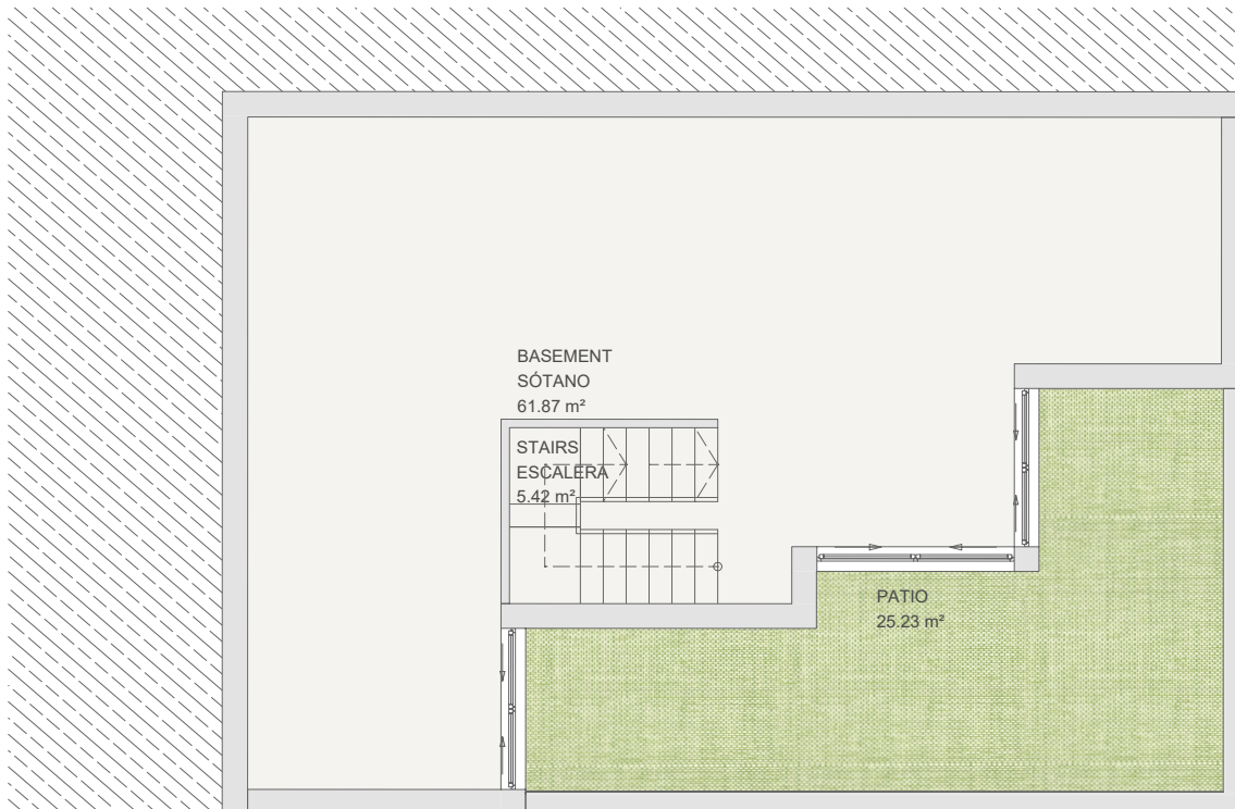
PLANTA SÓTANO
