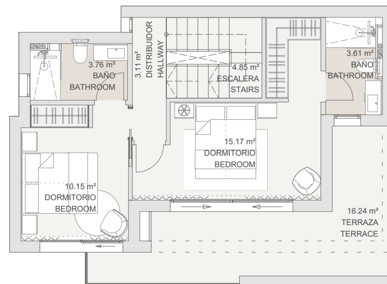
PLANTA PRIMERA
