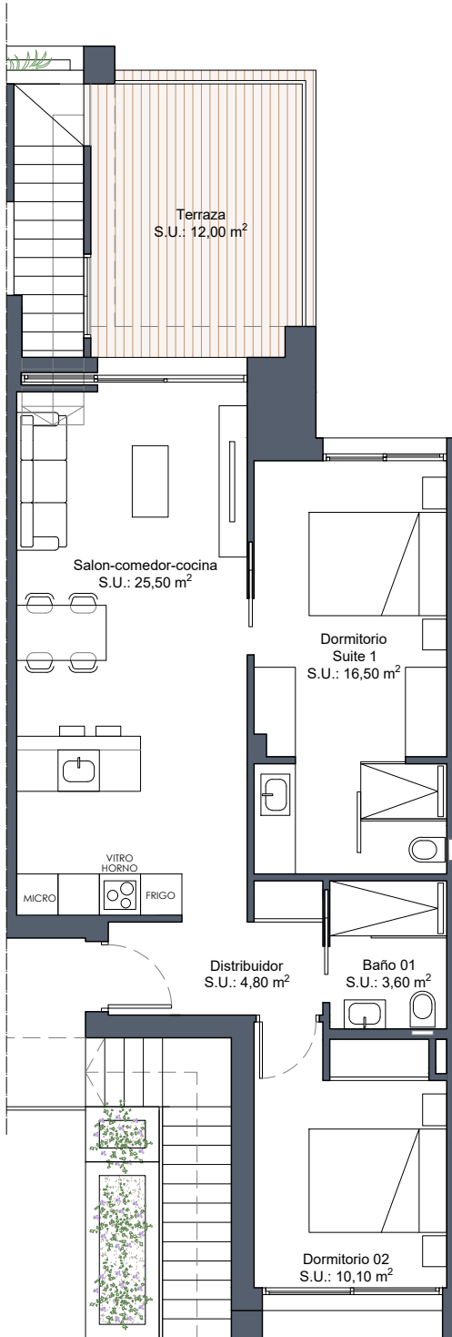
Planta primera
