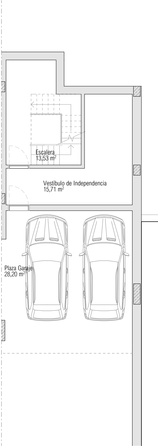
PLANTA SÓTANO
