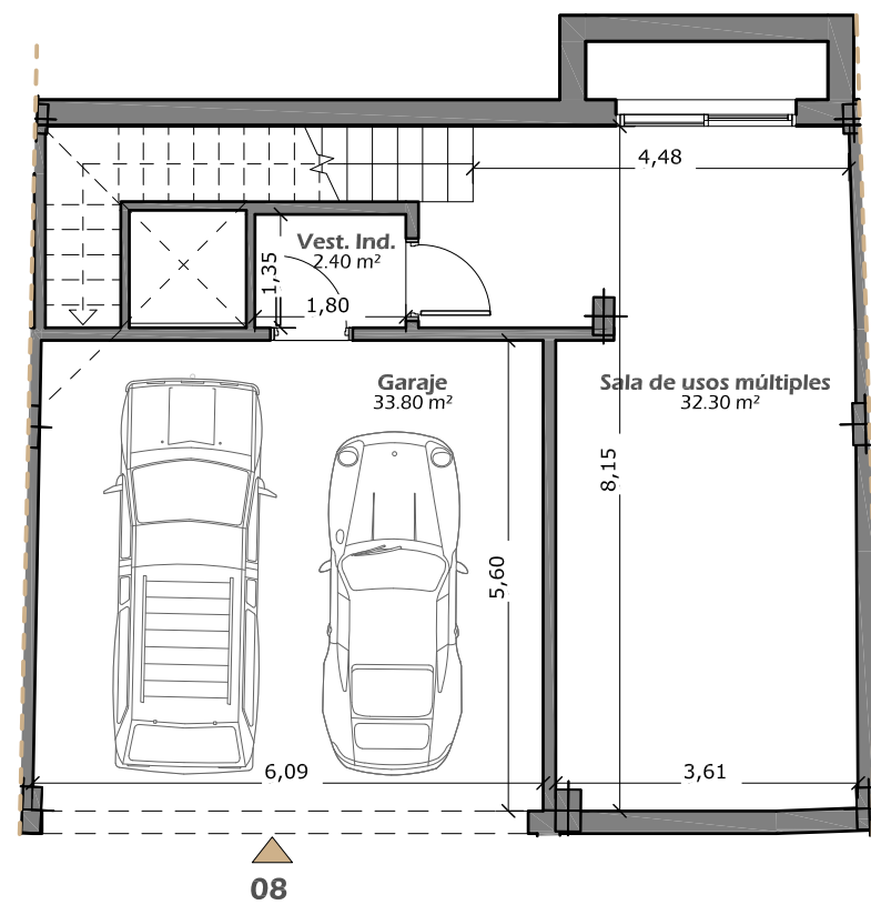
Planta Sótano
