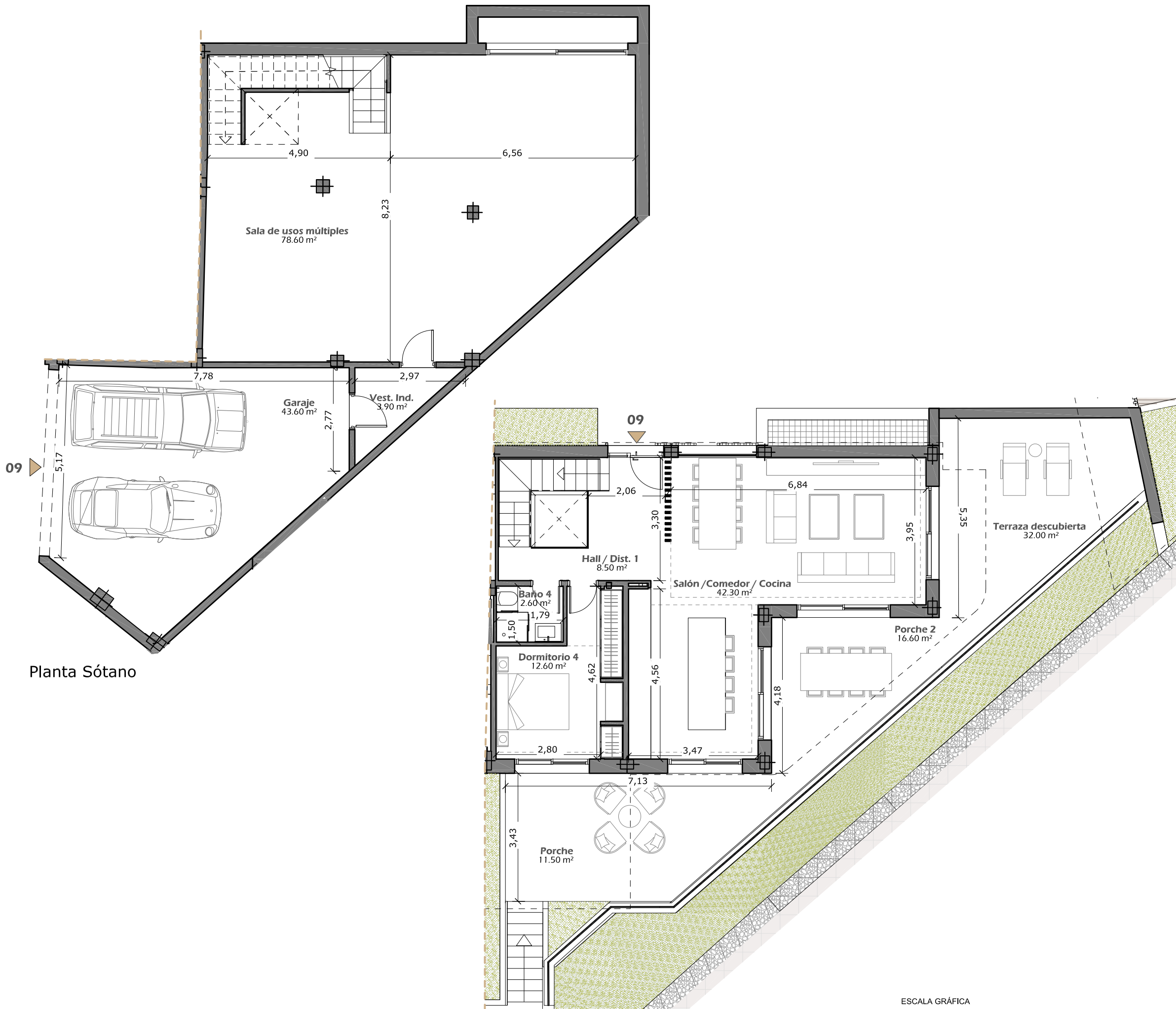
Planta Baja
