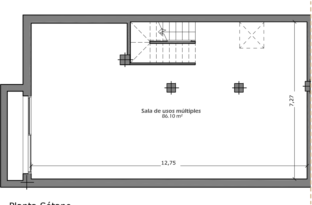
Planta Sótano
