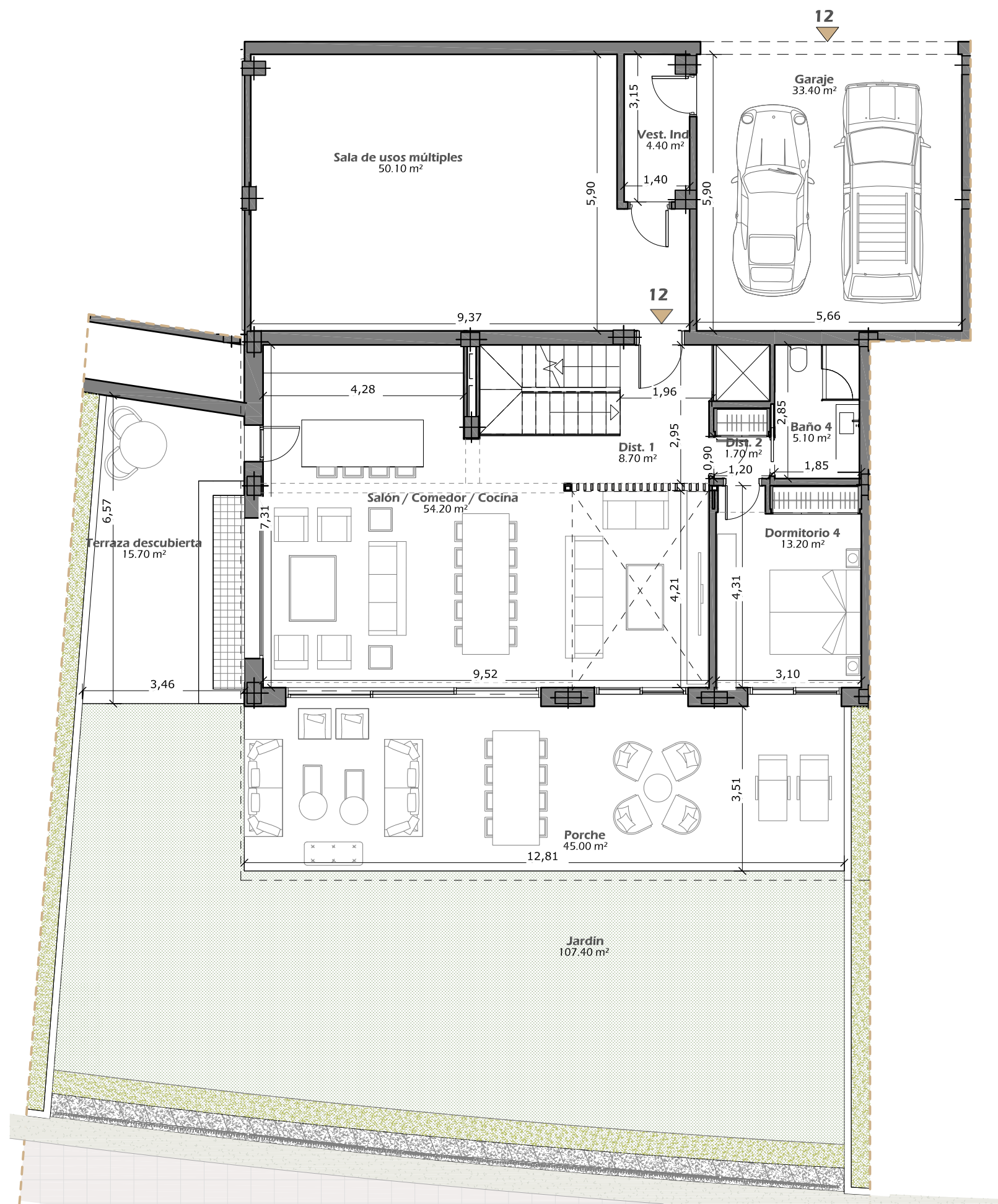
Planta Baja
