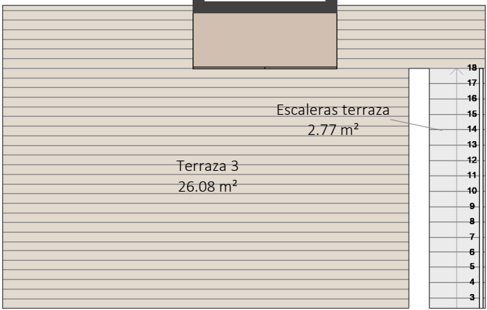
Planta Segunda / SECOND FLOOR
