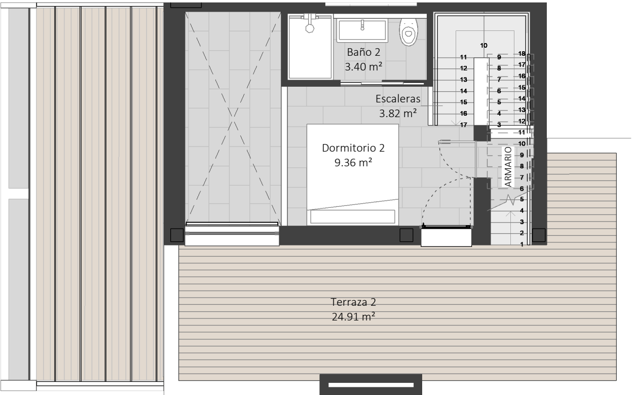
Planta Primera / FIRST FLOOR
