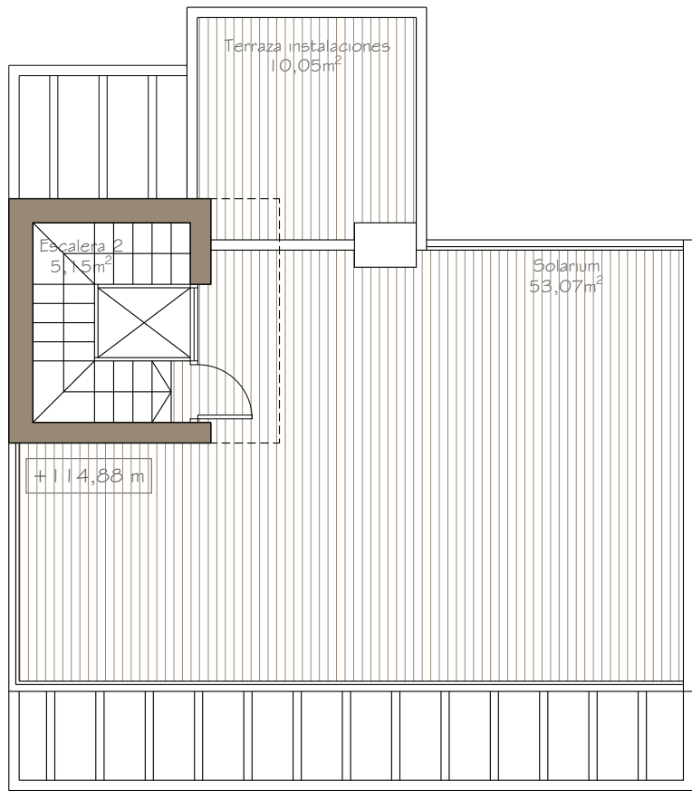
PLANTA CASTILLETE
