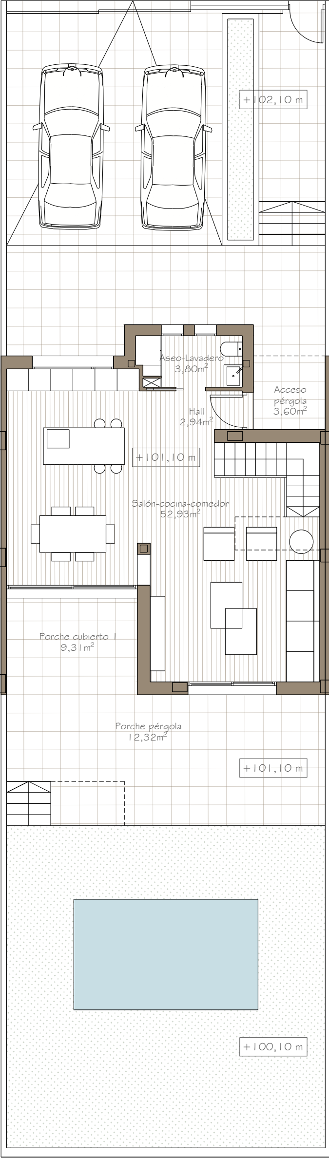
PLANTA BAJA
