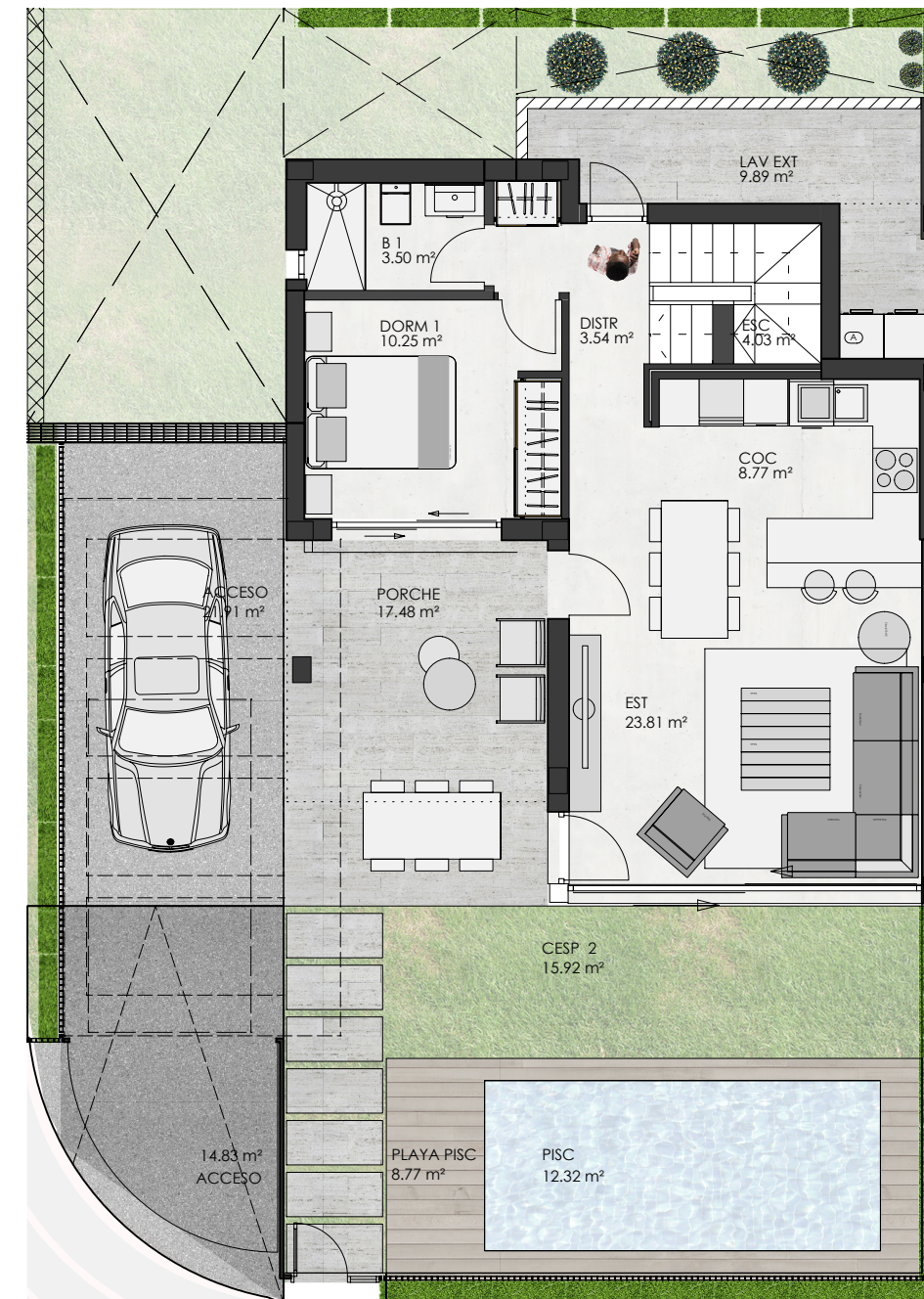
Planta Baja
