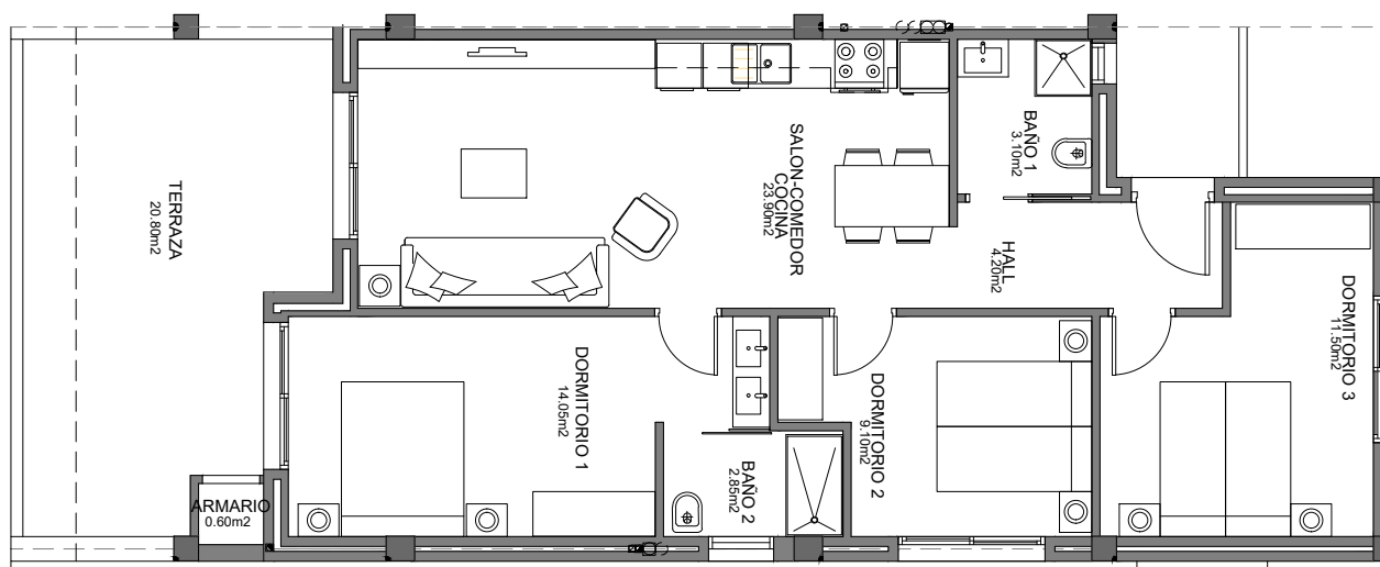
Planta Primera
