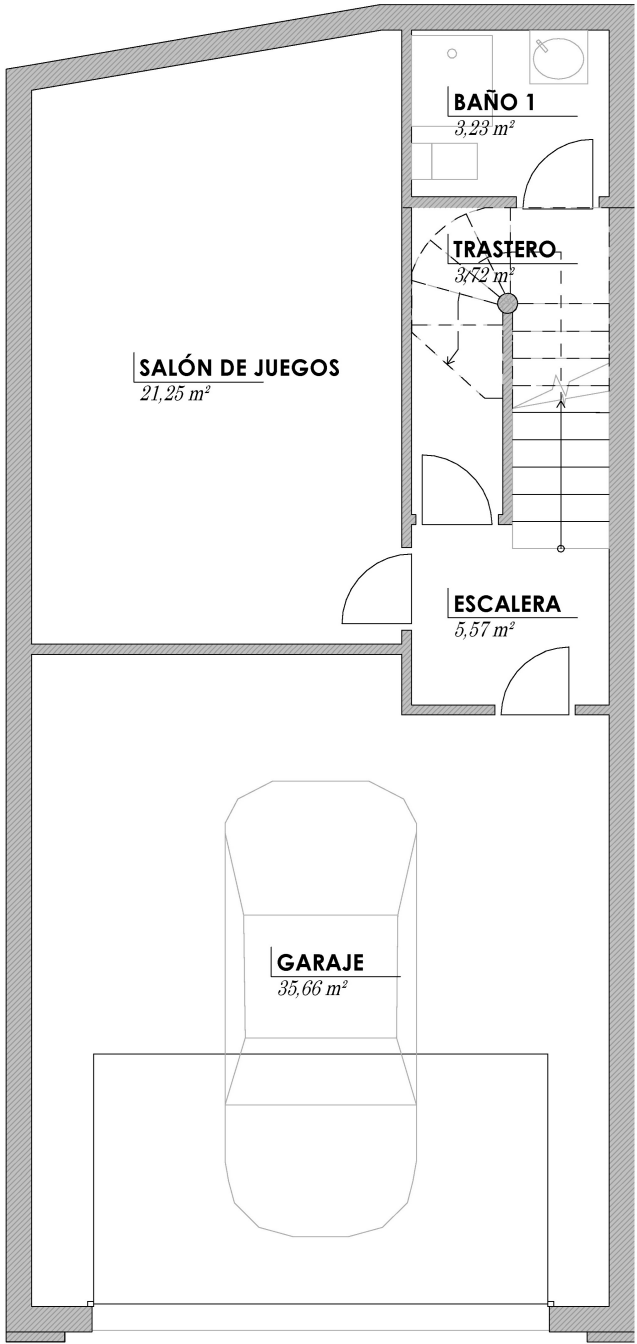
PLANTA SÓTANO
