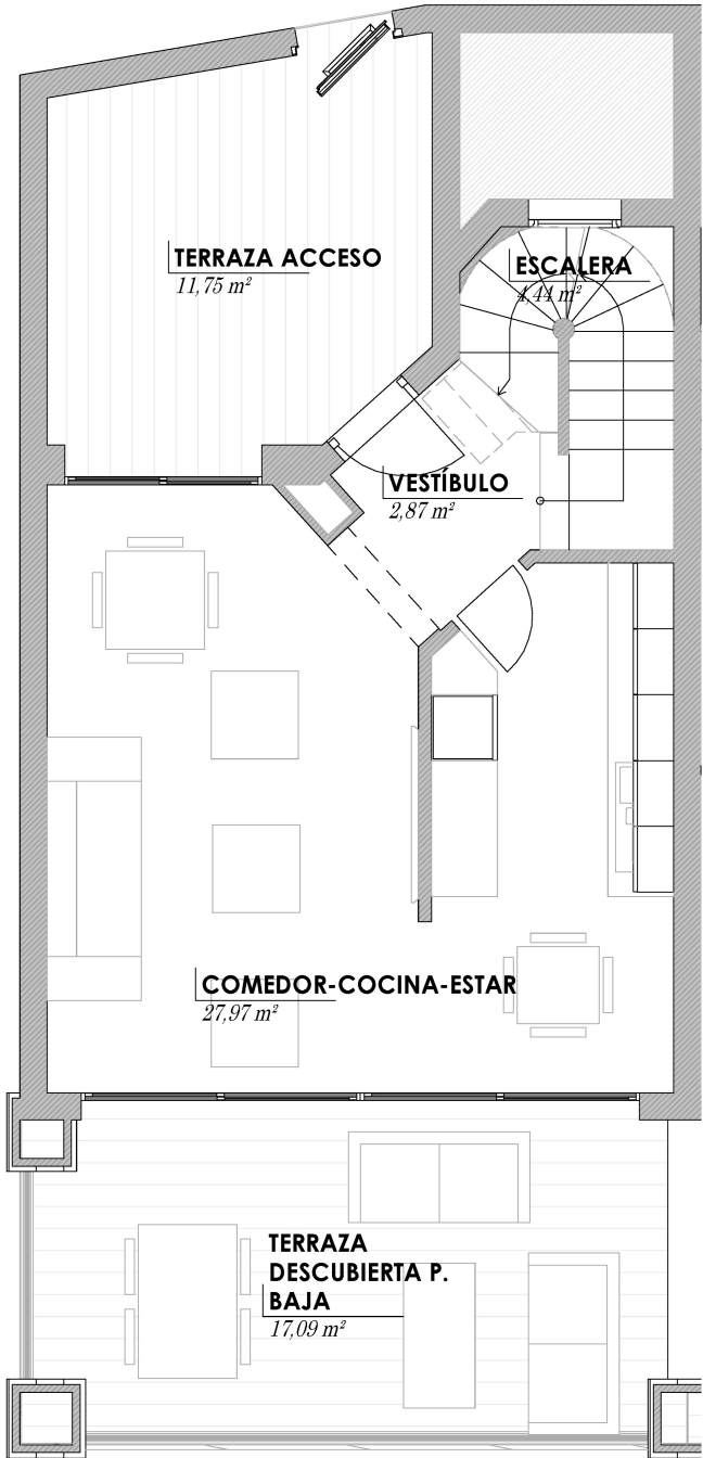
PLANTA BAJA
