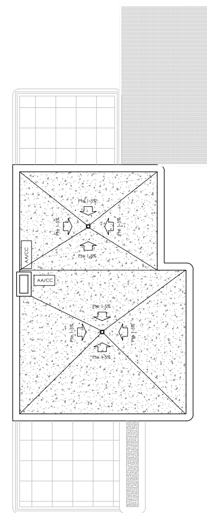
PLANTA CUBIERTA
