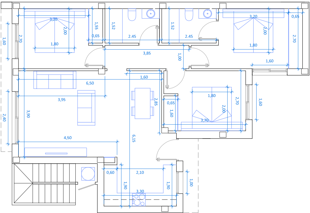
PLANTA MODELO B'
