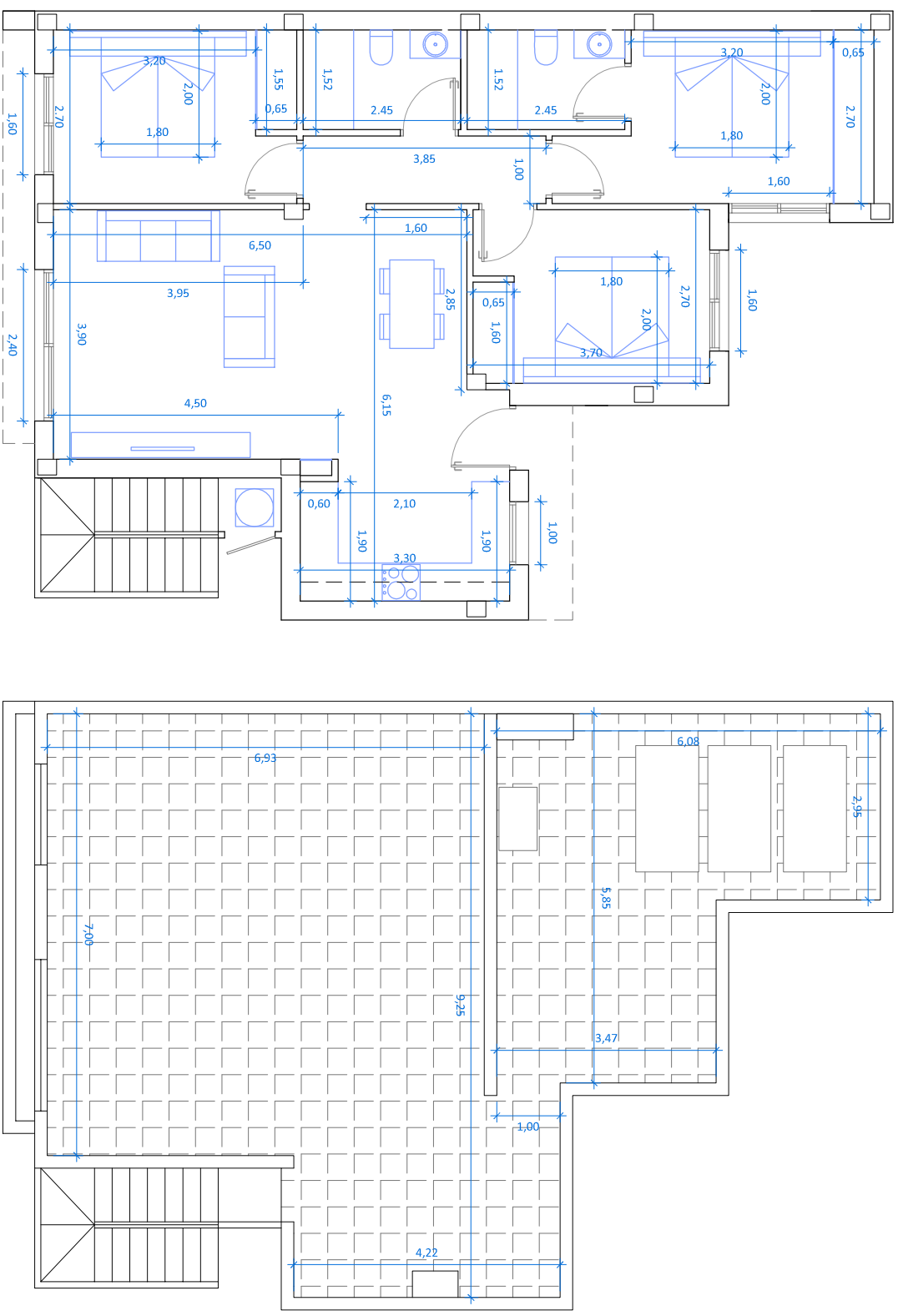
SOLARIUM MODELO B'
