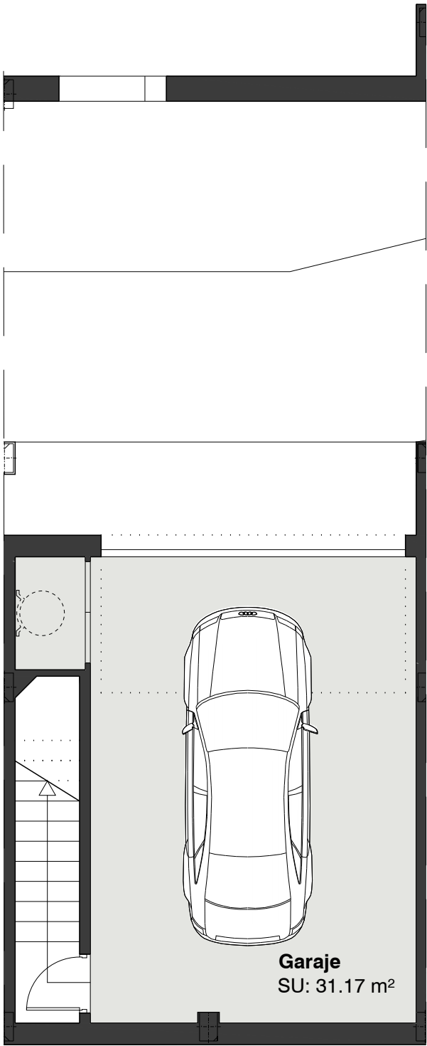
Planta sótano
