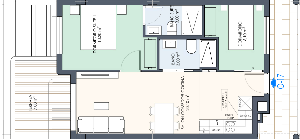
PLANTA PRIMERA
