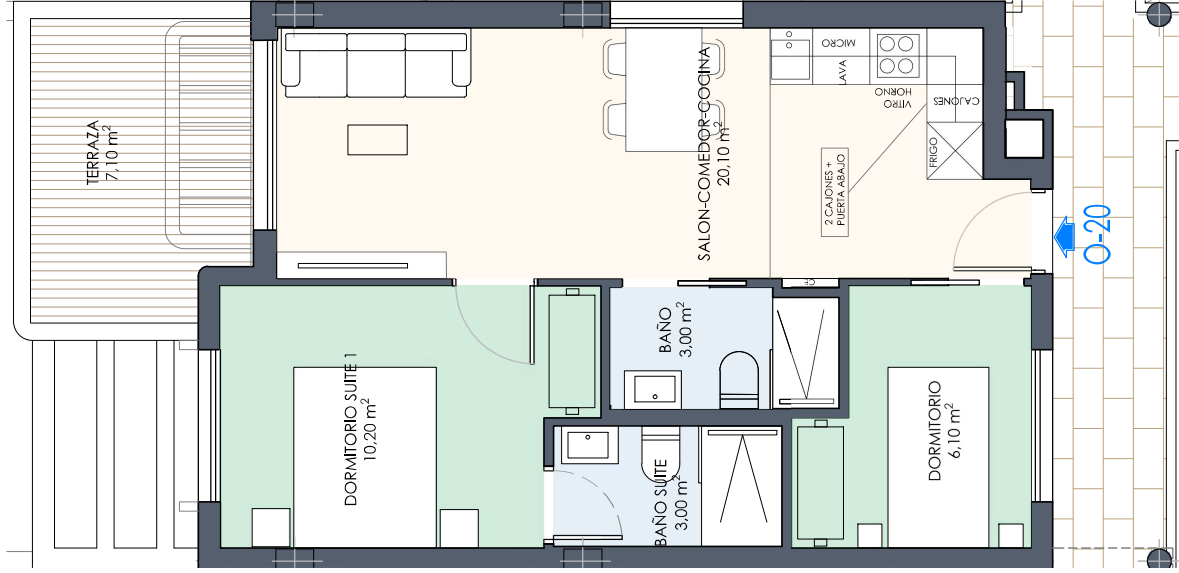
PLANTA PRIMERA
