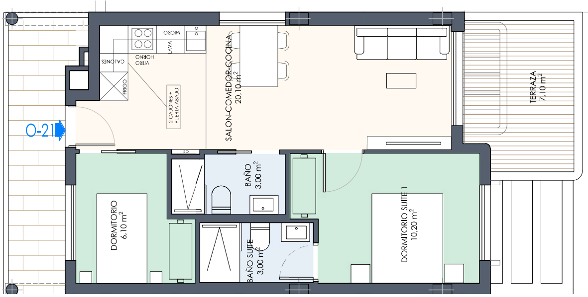
PLANTA PRIMERA
