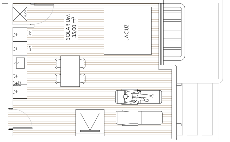
PLANTA SOLARIUM
