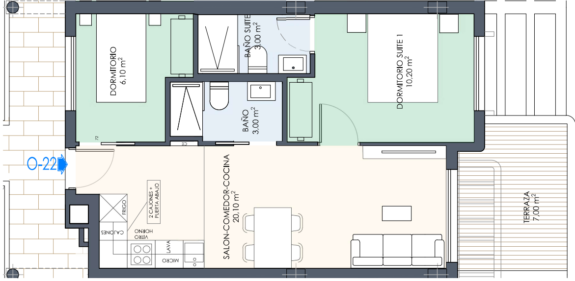
PLANTA PRIMERA
