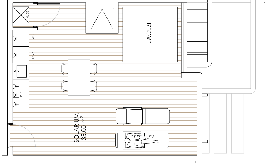
PLANTA SOLARIUM
