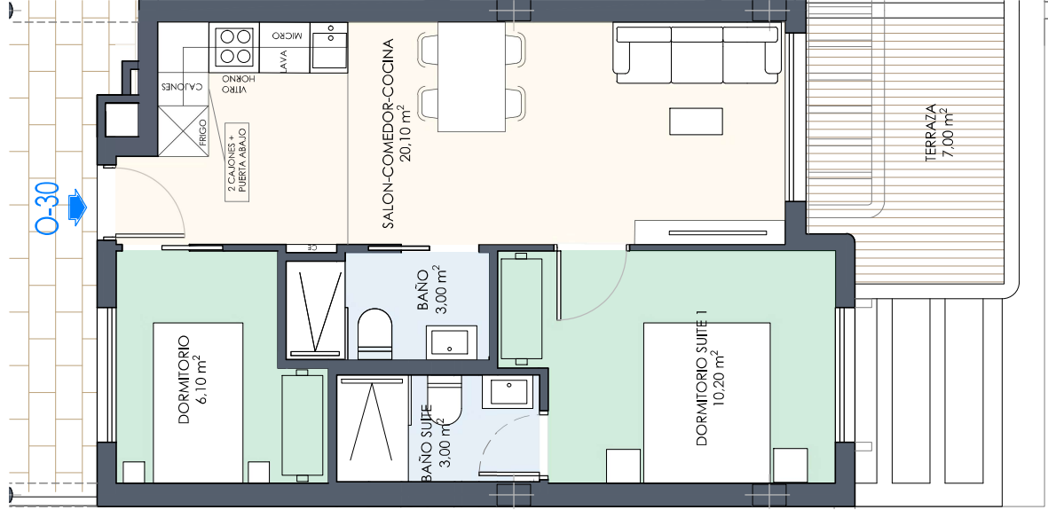
PLANTA PRIMERA
