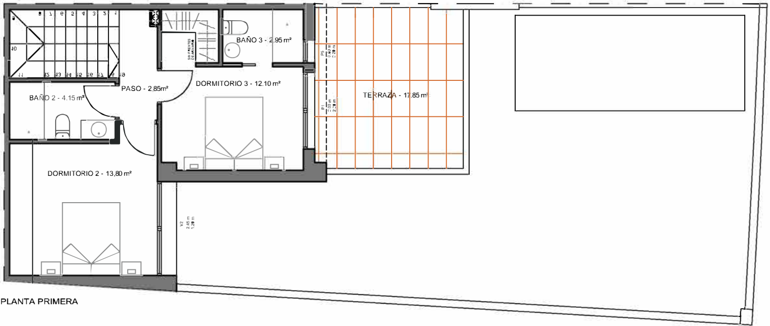
PLANTA SOLARIUM
