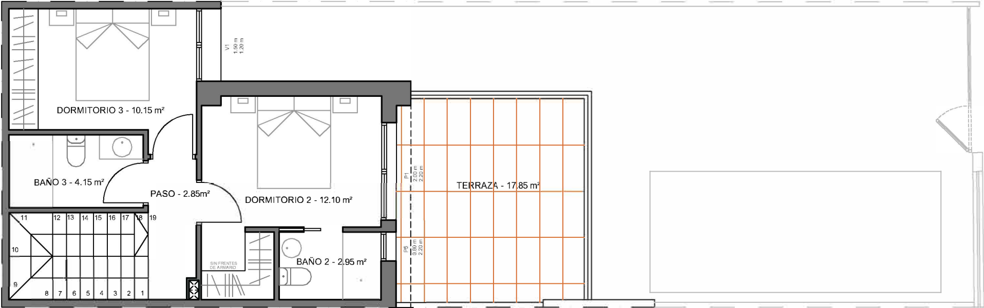
PLANTA PRIMERA
