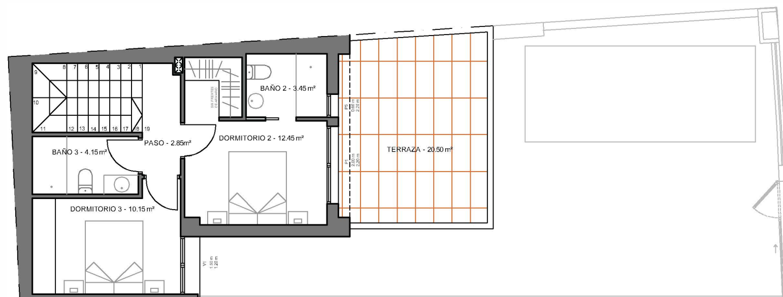
PLANTA PRIMERA
