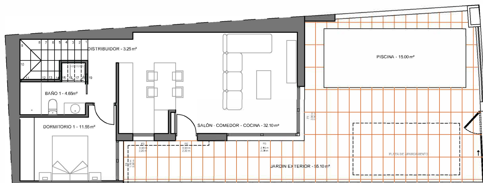
PLANTA BAJA
