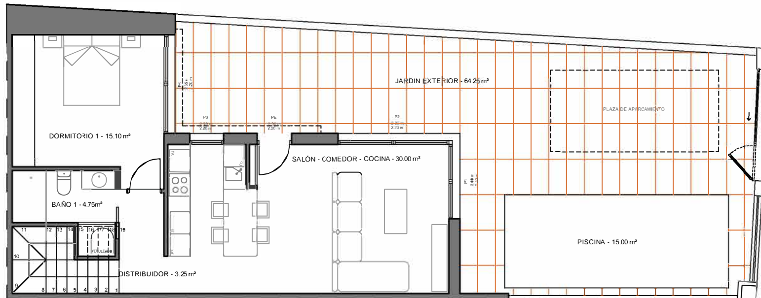
PLANTA BAJA
