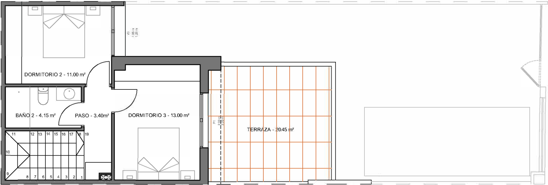
PLANTA PRIMERA
