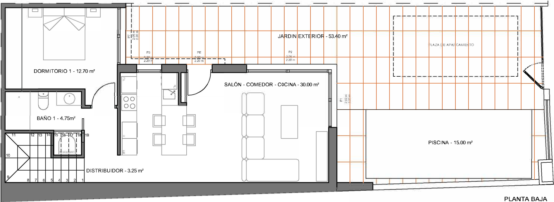
PLANTA BAJA
