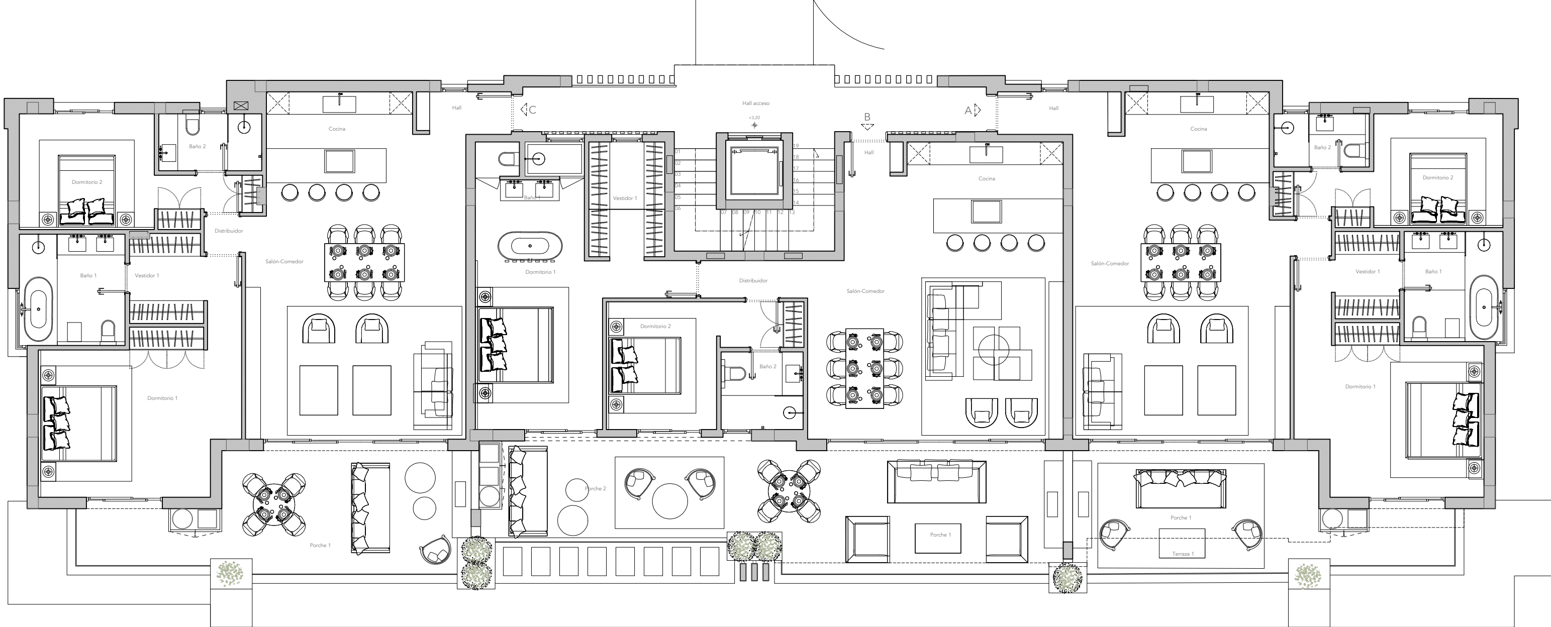
PLANTA PRIMERA_BLOQ. 1
