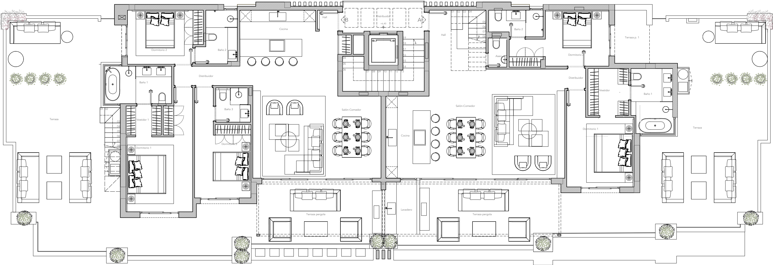
PLANTA SEGUNDA_BLOQ. 1
