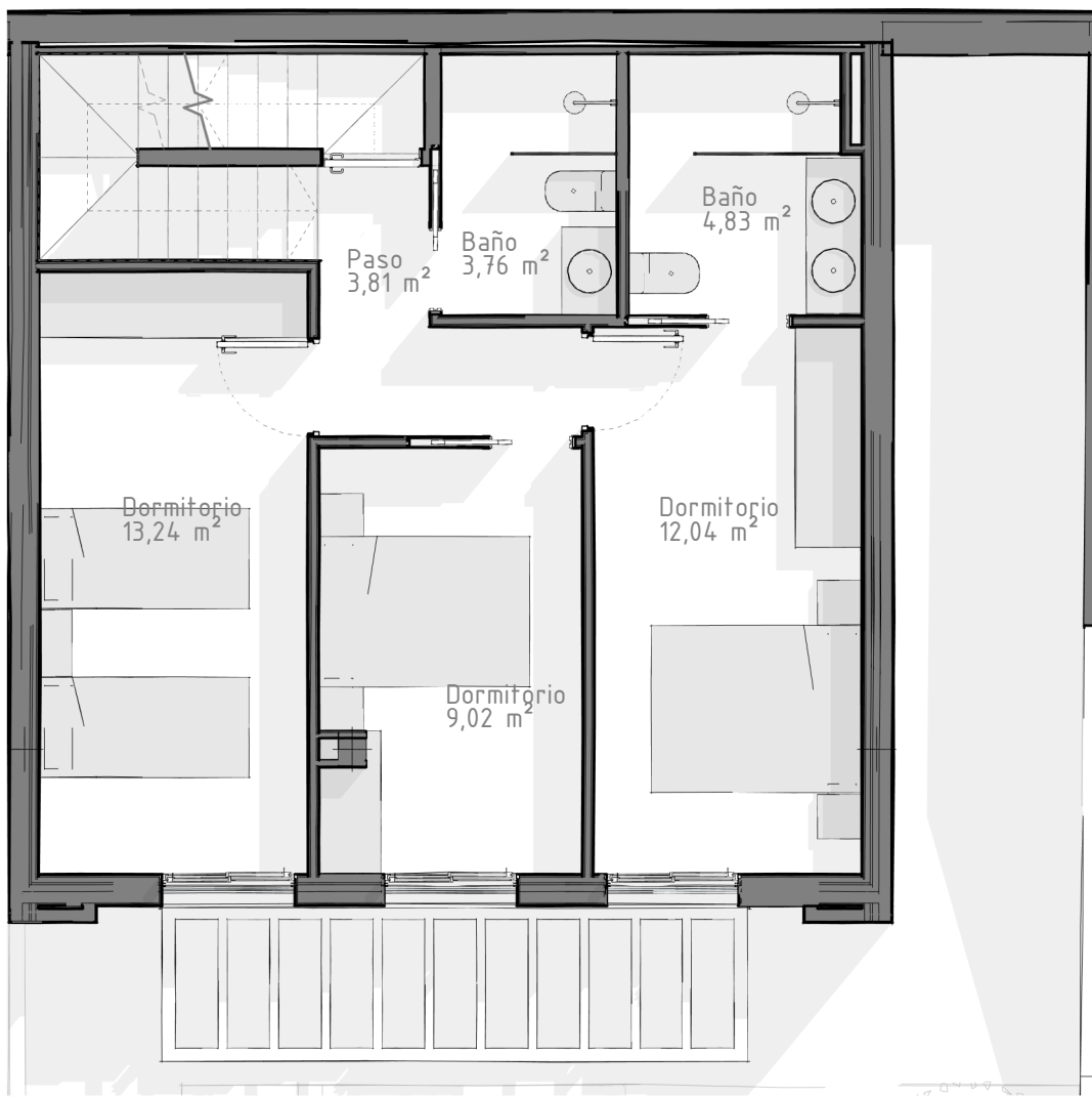
1.Viv. Unifamiliar. Planta 1ª
