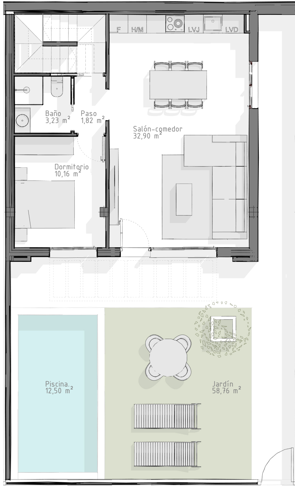
2.Viv. Unifamiliar. Planta baja
