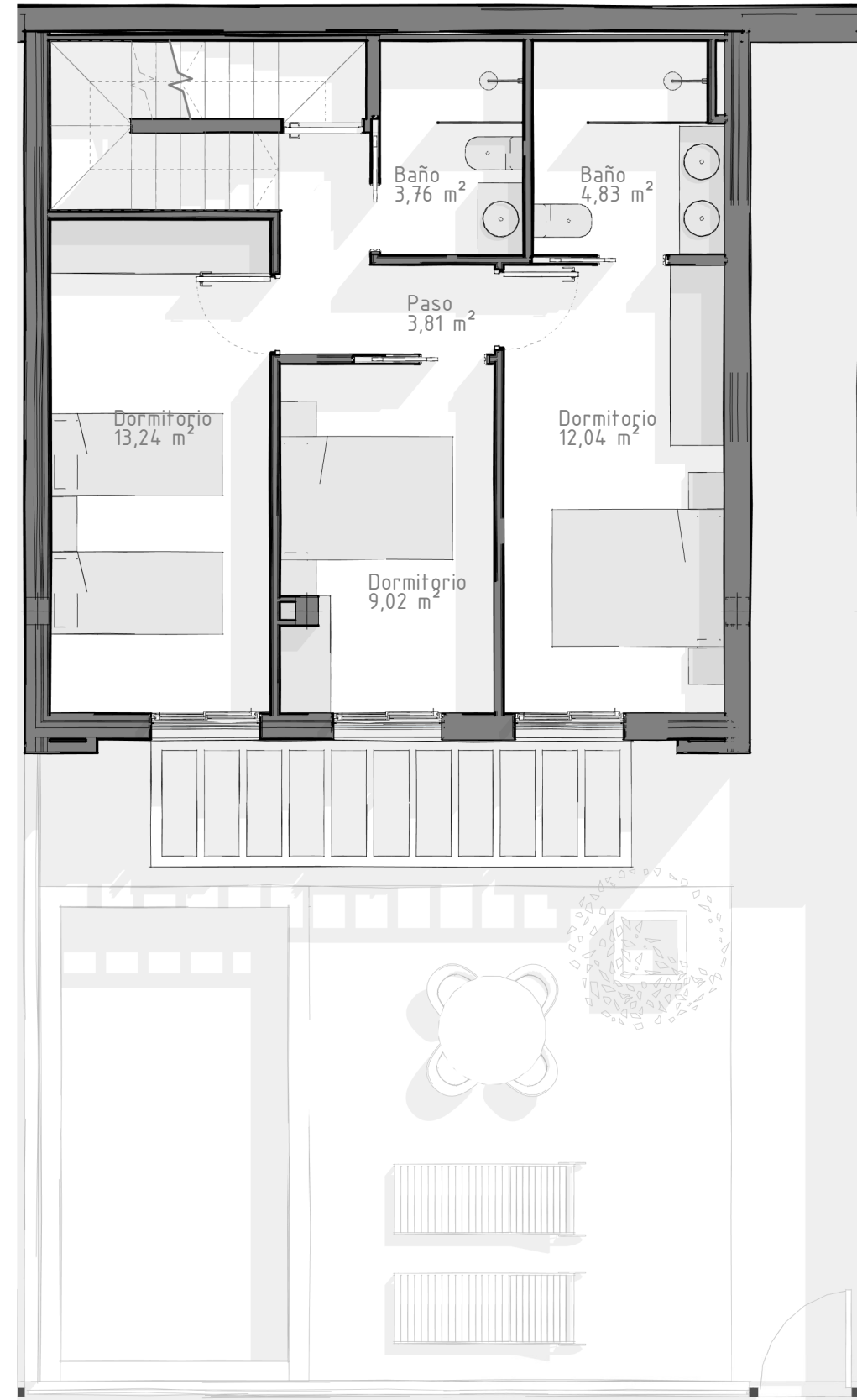
2.Viv. Unifamiliar. Planta 1ª
