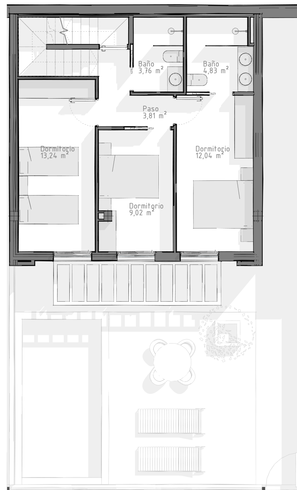
7.Viv. Unifamiliar. Planta 1ª
