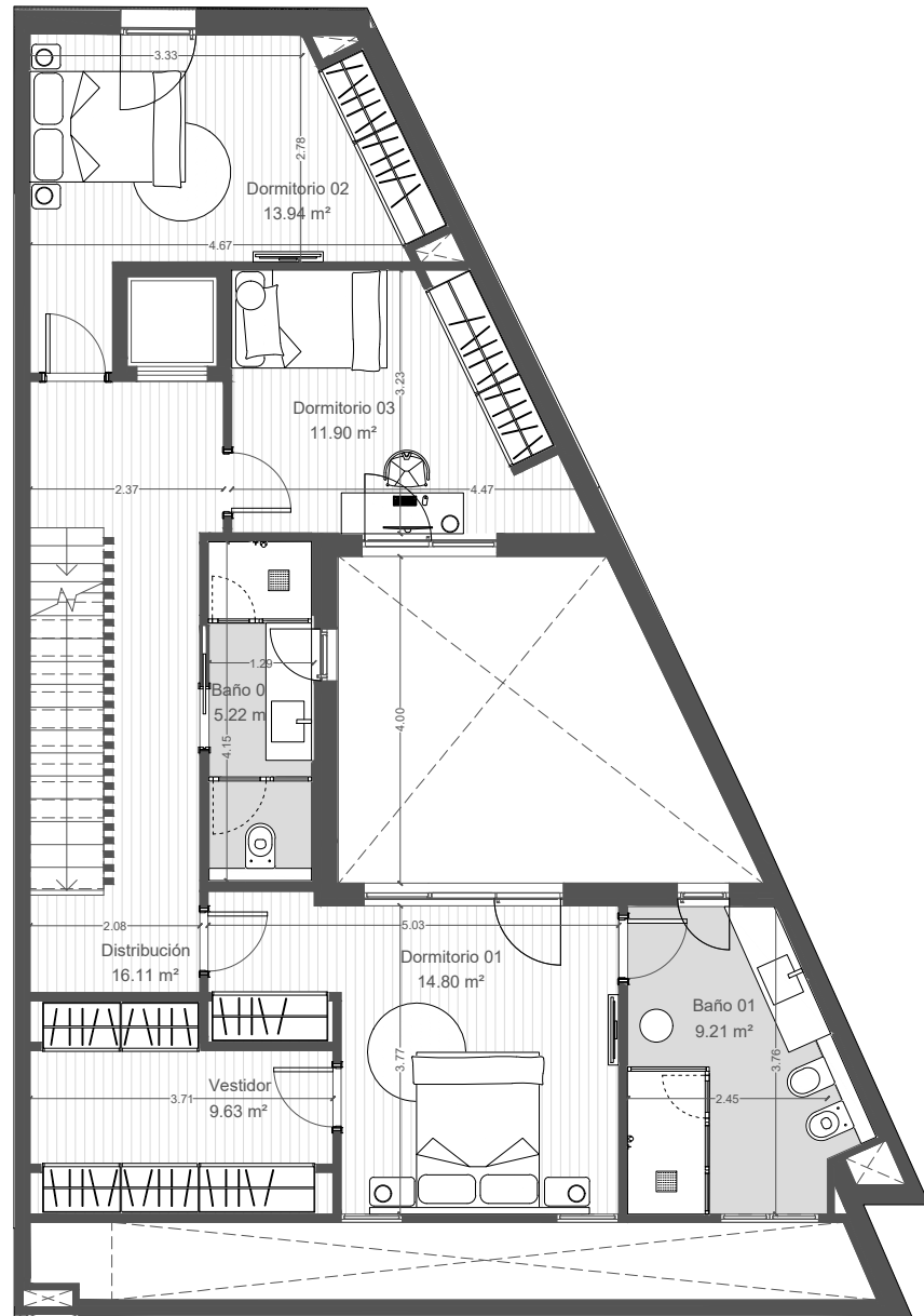
Planta Primera
