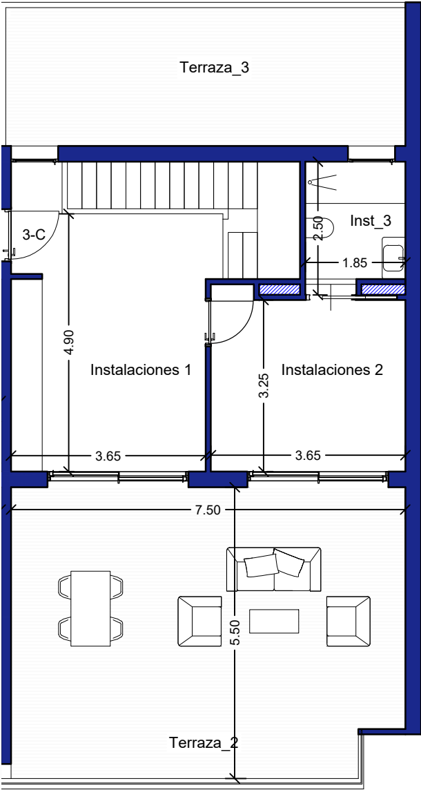
PLANTA BAJO CUBIERTA
