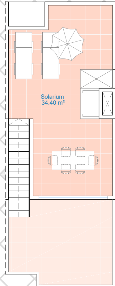
PLANTA SOLARIUM
