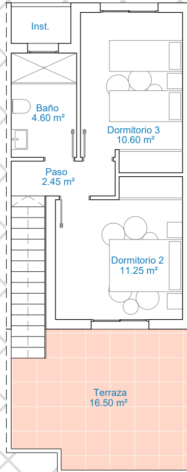
PLANTA PRIMERA
