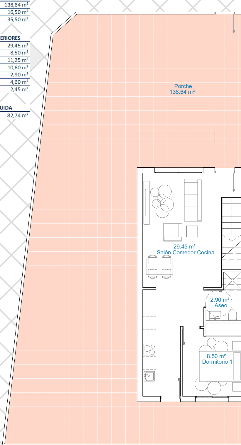
PLANTA BAJA
