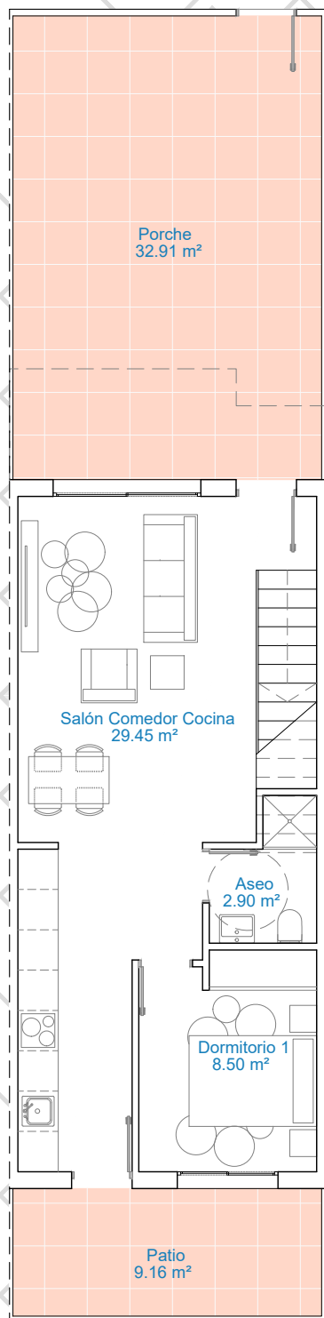
PLANTA BAJA
